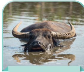
c. bivolul;
